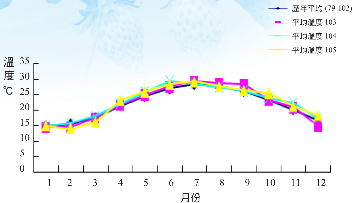
圖 73、月平均溫度變化（歷年：79-102 年之平均）。
