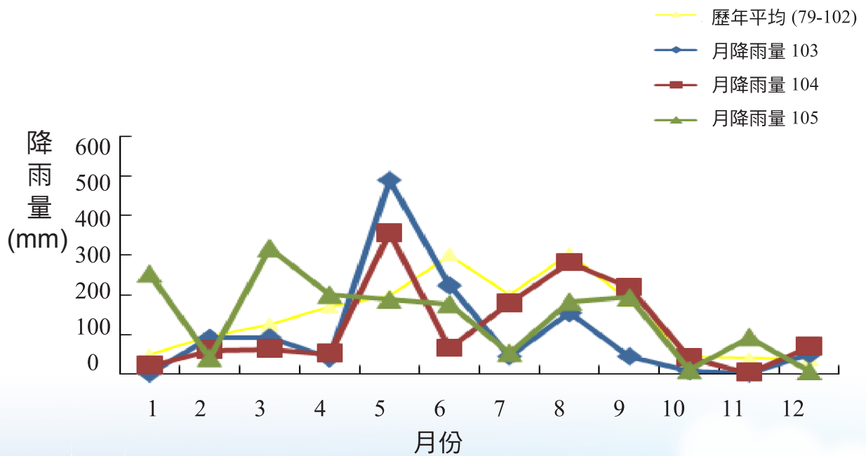
圖 76、月降雨量之變化 (歷年：79-102 年月平均)。
