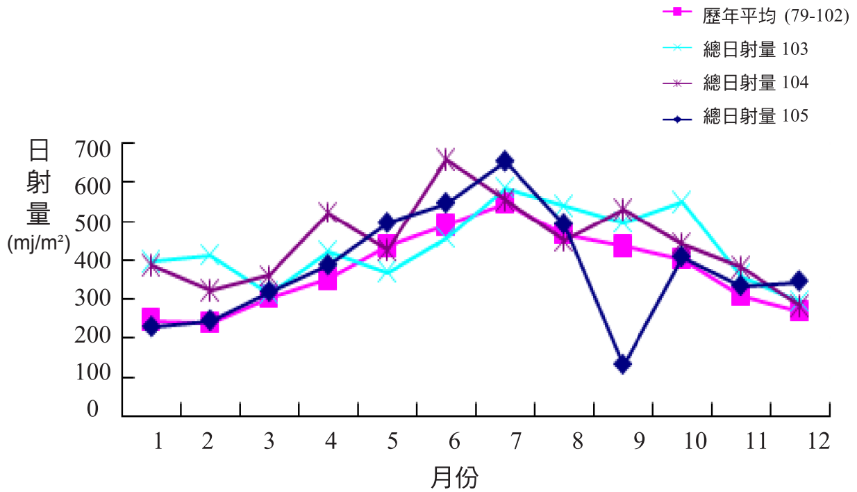
圖 75、月總日射量之變化 (歷年：79-102 年月平均)。
