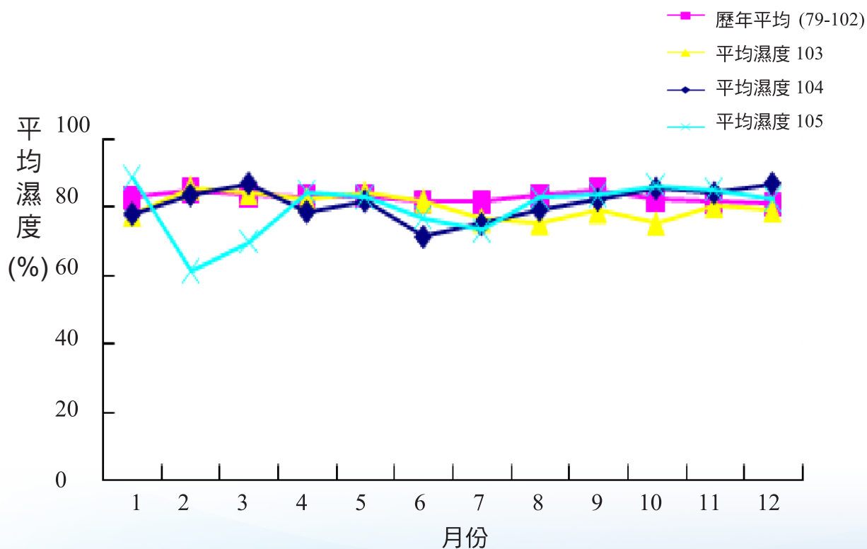
圖 74、月平均濕度變化（歷年：79-102 年之平均）。
